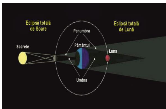
Fig.2 – Schema formării eclipselor de Soare și Lună
