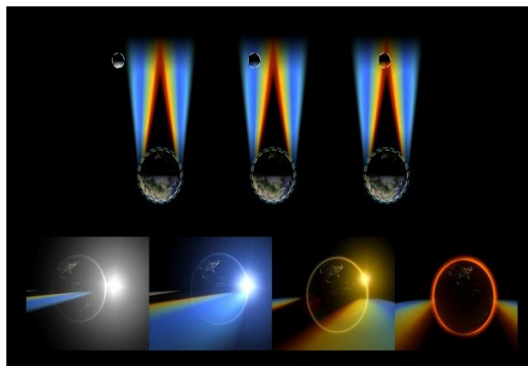
Fig.4 – Refracția luminii prin atmosfera terestră
