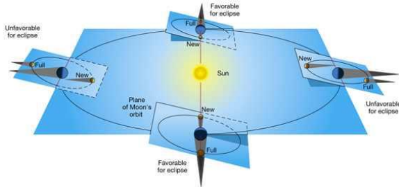
Fig.1- Planul orbitei Lunii cu planul orbitei Pământului
